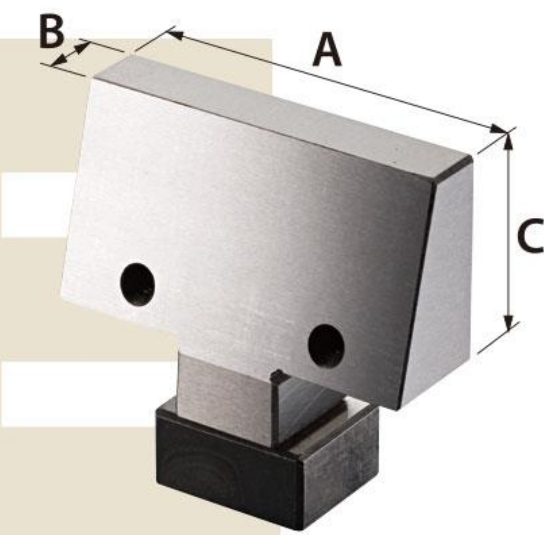
Комплект передвжных насадок с односторонним скосом кромки
