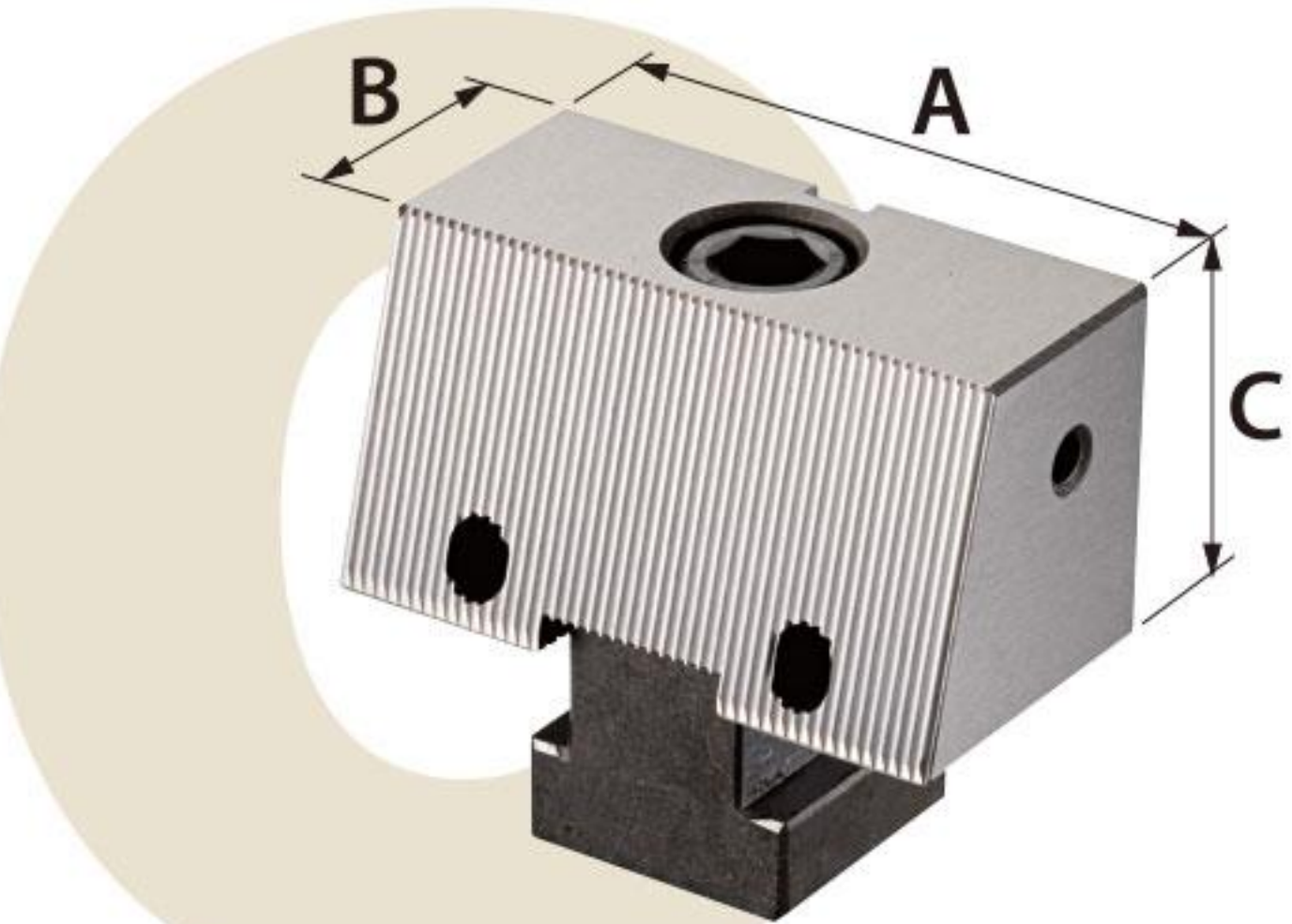
Комплект фиксированных насадок с односторонним скосом кромки
